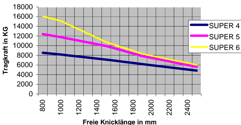
Tragkraftdiagramm der Rahmen
